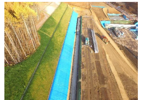
排水フリーム設置状況 （施工中）
